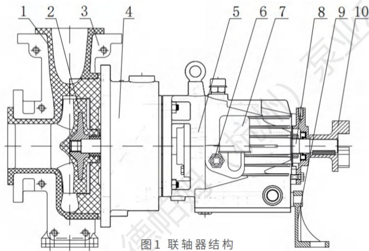
图1 联轴器结构
