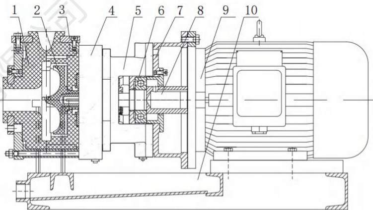
图2 直连式结构
